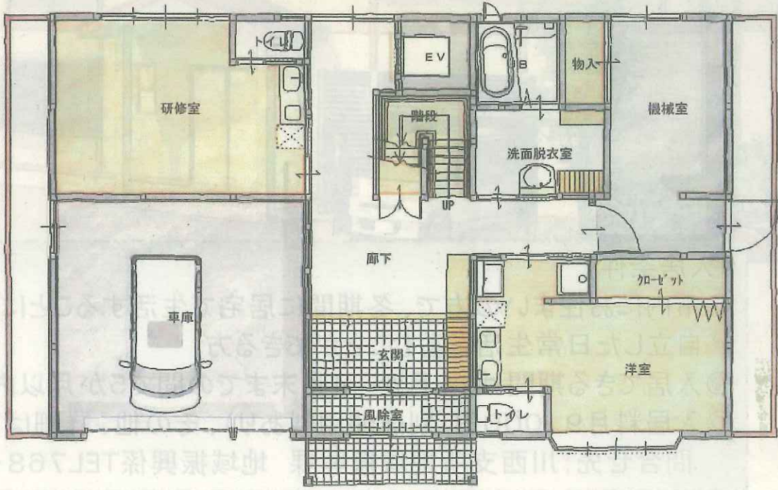
1階 平面
