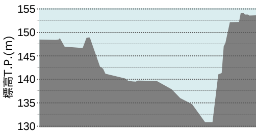
断面模式図
