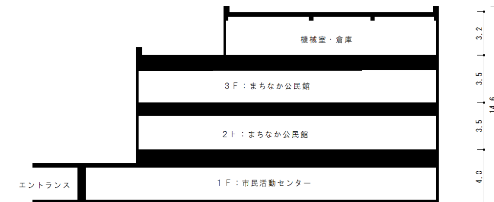
施設断面図
