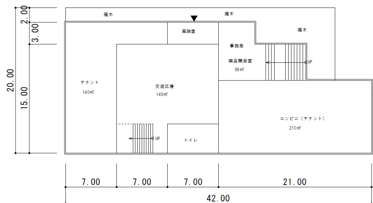
1階平面図
