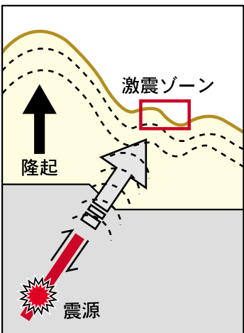
図2 震源と激震ゾーンの関係
