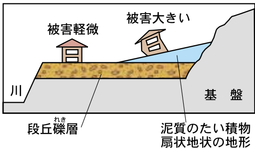
図3 段丘地形と建物被害
