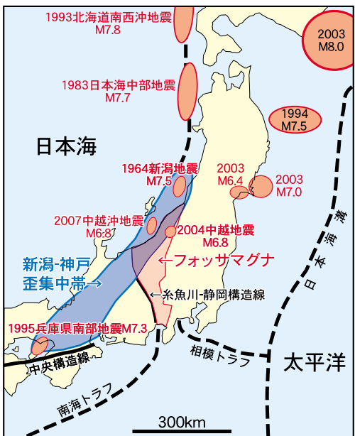
図1 フォッサマグナと新潟―神戸歪集中帯
