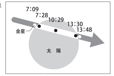
6月6日の金星日面通過イメージ
