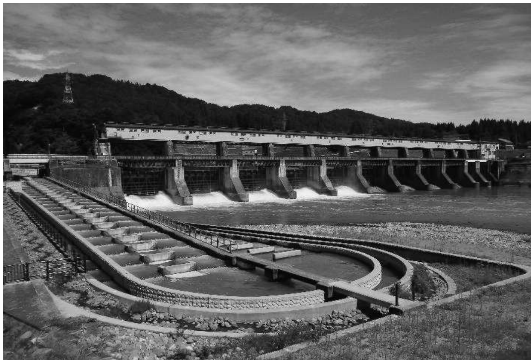
JR東日本信濃川発電所宮中取水ダム
