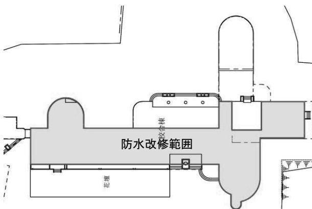
松代中学校校舎屋根防水改修工事平面図
