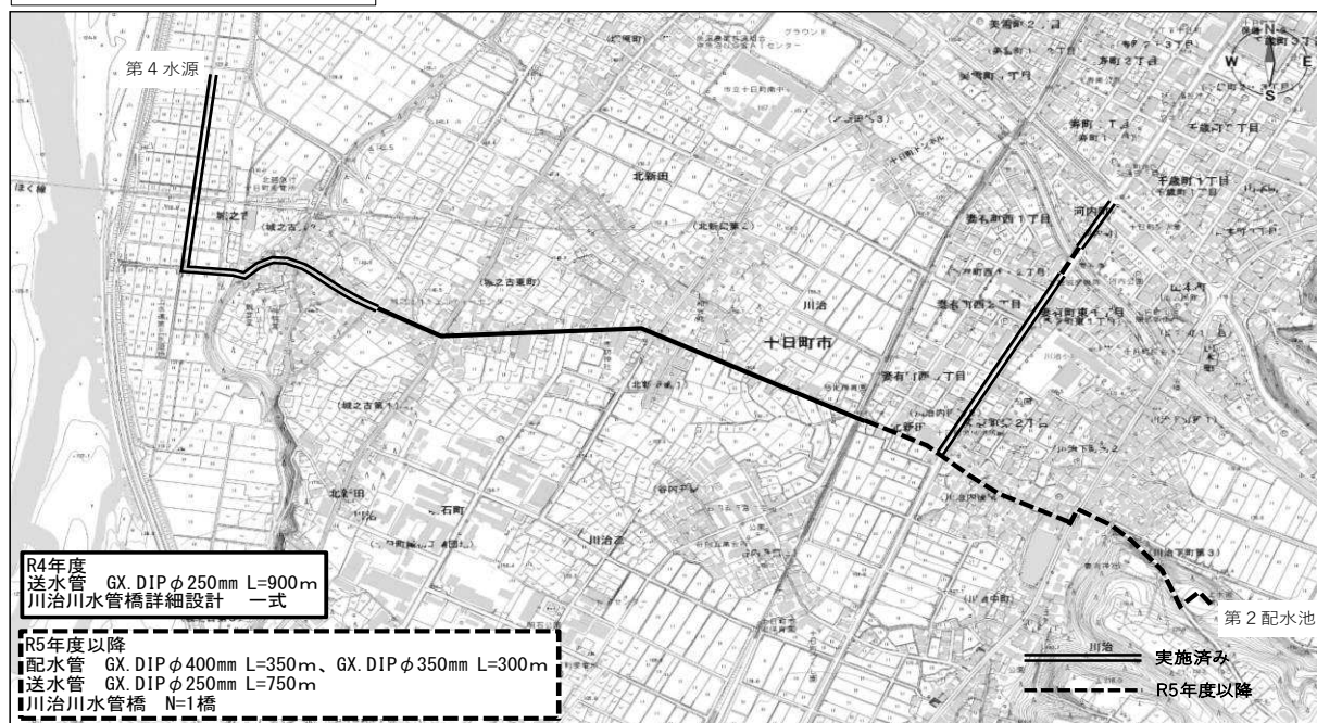
十日町第2配水系基幹管路耐震化事業
