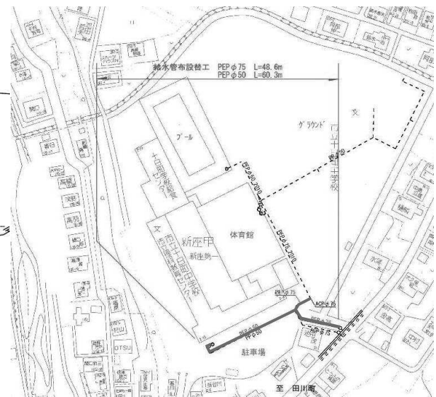
十日町中学校給水管布設替工事平面図
