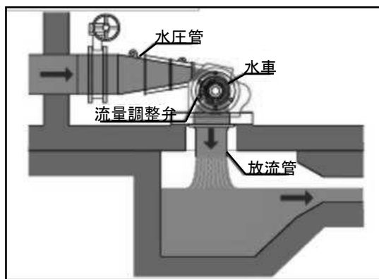
小水力発電検討箇所の取水口
