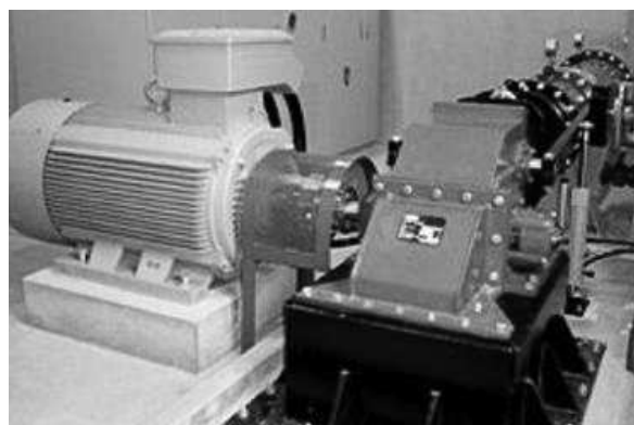
小水力発電の仕組みと設備
