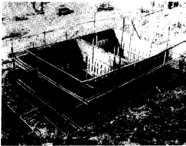
▲ 木落・寺ヶ崎簡水の配水池工事
