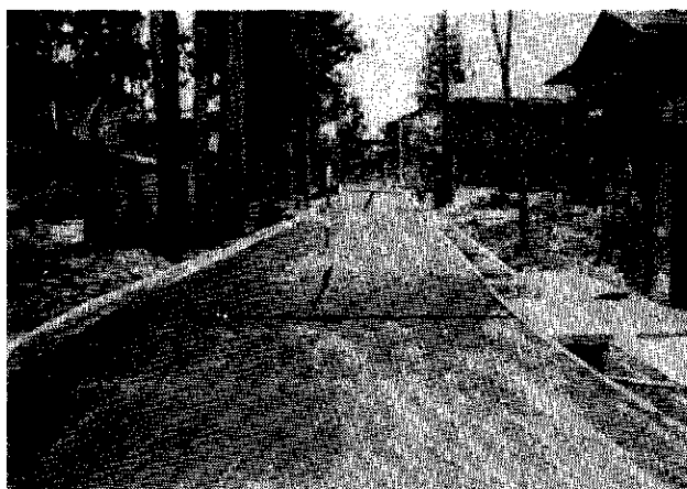
↑ 伊友裏町線 着手前 ↓ 伊友裏町線 完 成
