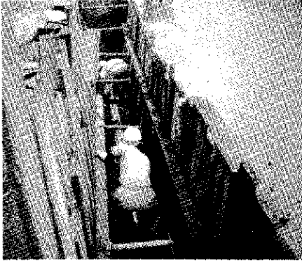
橘地区下水管路工事（仁田地区）
