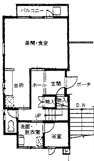
2階平面図
