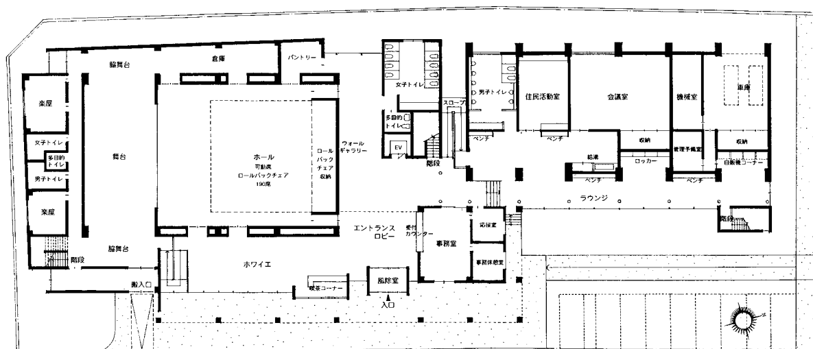
1階平面図
