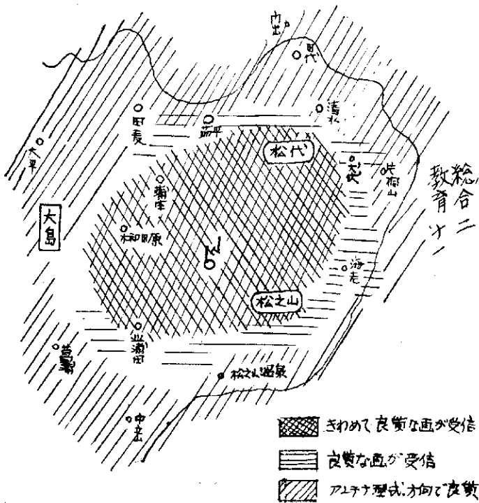
NHK松代テレビジョン受信状況予想図
