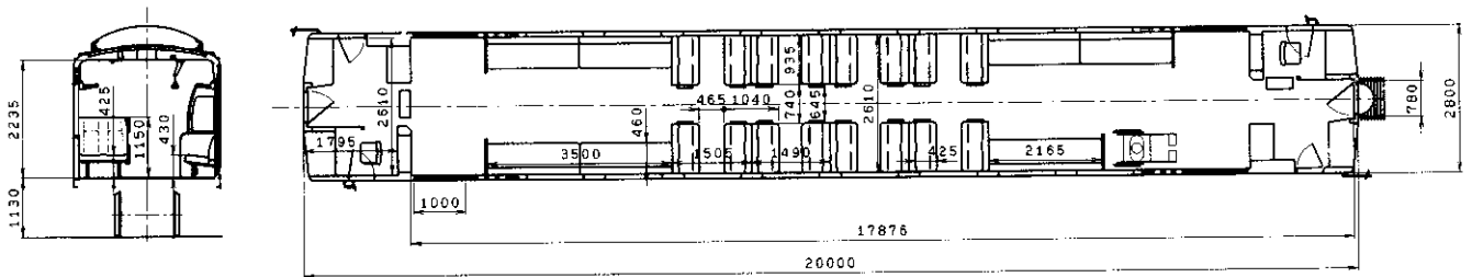
車体寸法図 (単位mm)
