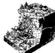
がけ崩れ
