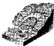
地すべり
