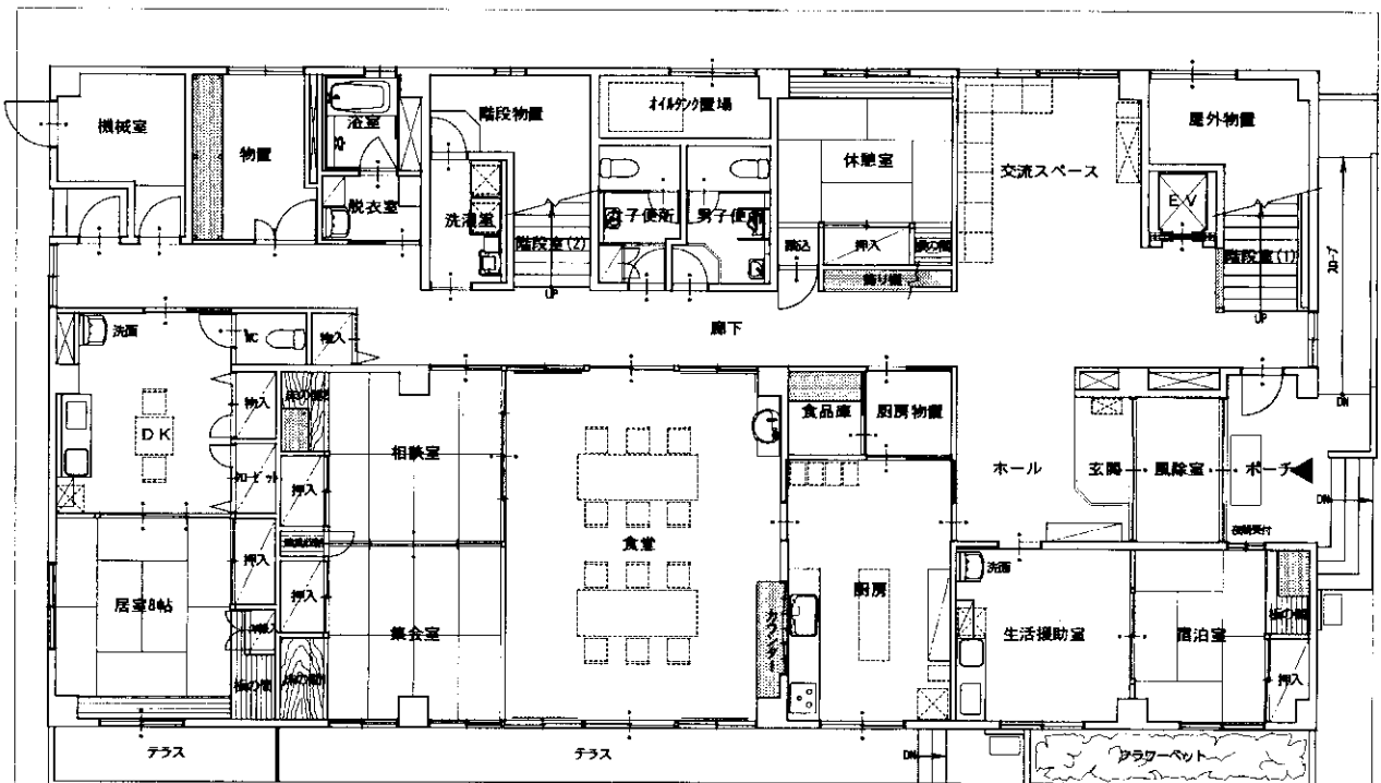
1階平面図
