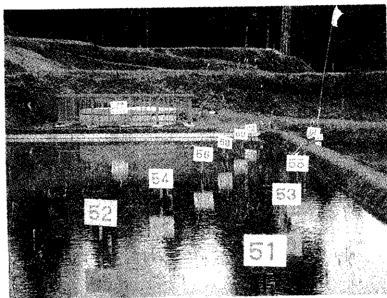
威力を発揮する集水井と鋼管杭 鋼管杭は番号札の下に打ち込まれています
