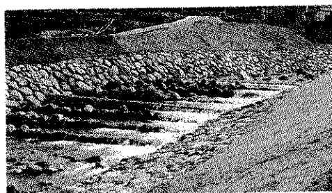
渋海川の巨石を利用した護岸
