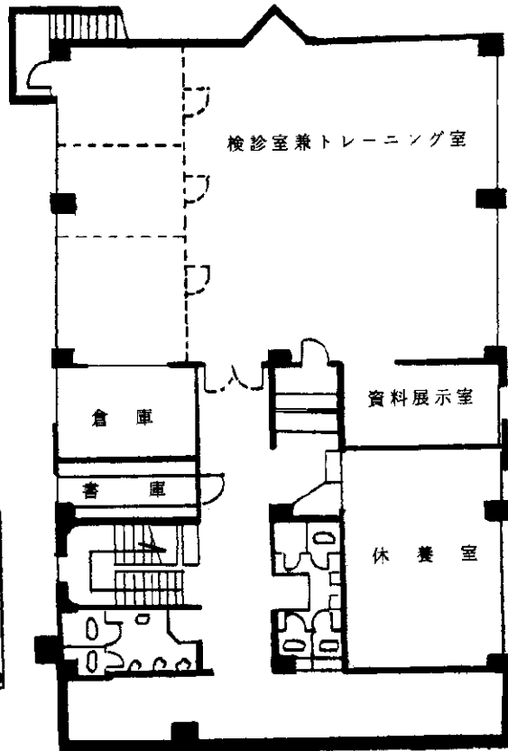
二階平面図
