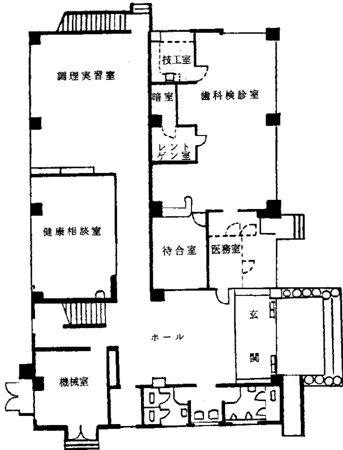
一階平面図
