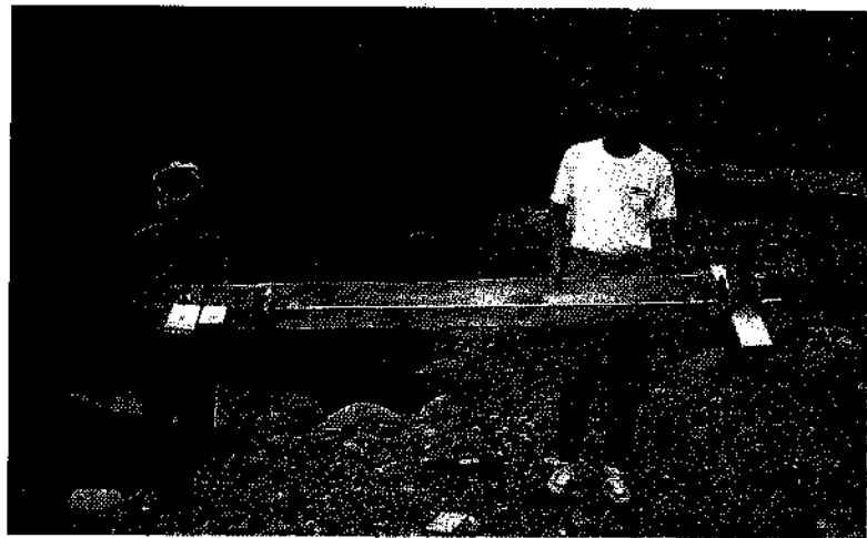
自作の水力発電機を手にする山本忠君と山本恭史君
