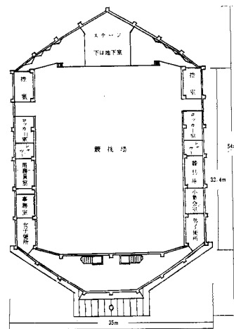
市民体育館 1階平面図
