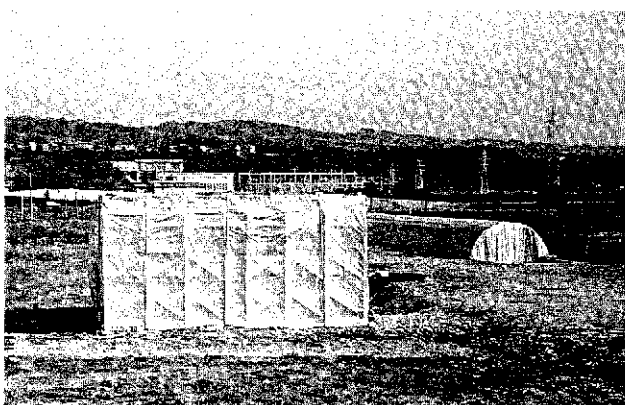
下水処理センターで行われている雪保存利用実験
