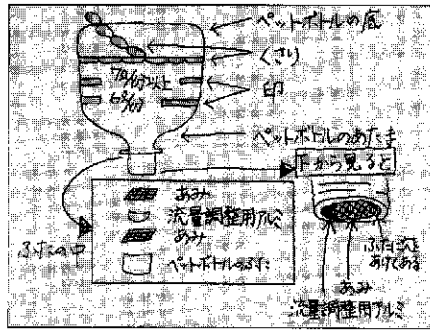
節水用流量計の構造図
